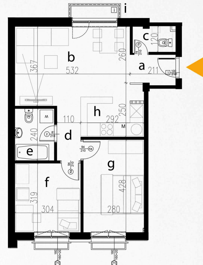
osnova stana sa dimenzijama
